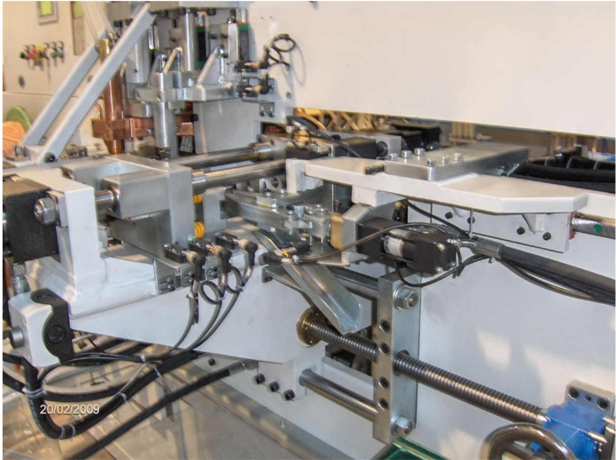
VISTA DEL SISTEMA TRAINO E DEL TAGLIO.
